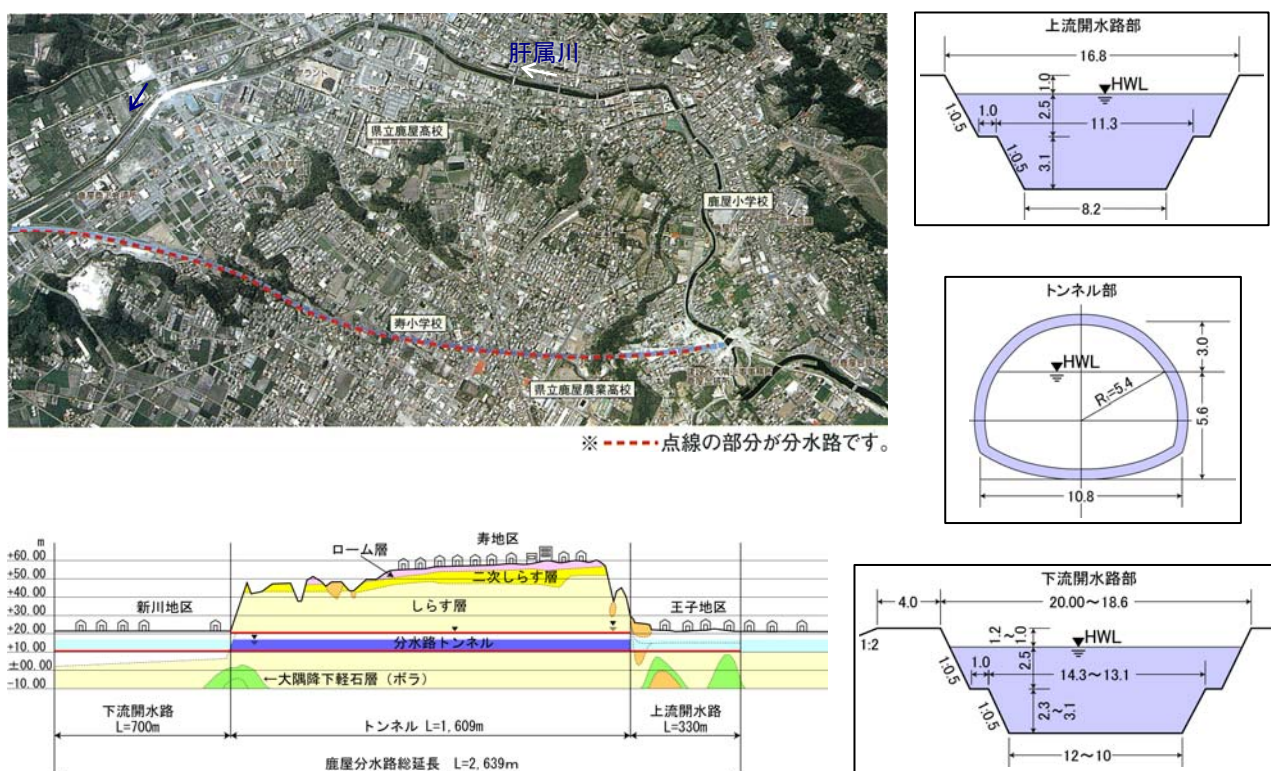
図 1.2.3 鹿屋分水路概要図
