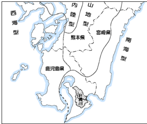
図 1.1.8 九州南部の気候区分 出典) 福岡の気象百年
